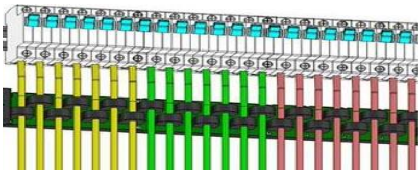
图 2.3.1 HC-31CA 典型接线示意图
