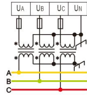
图 2.3.5 三相三线3PT接入
