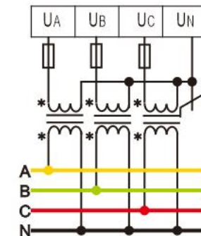
图 2.3.4 三相四线3PT接入
