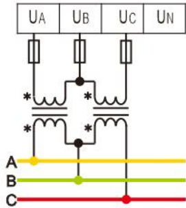
图 2.3.6 三相三线2PT接入
