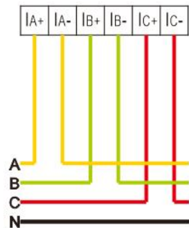
图 2.3.7 三相电流直接接入
