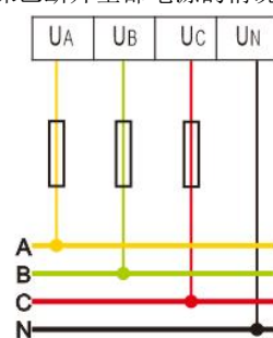
图 2.3.2 三相四线直接接入
