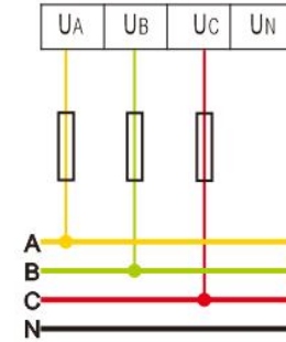
图 2.3.3 三相三线直接接入
