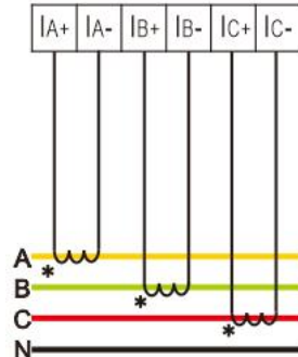
图 2.3.8 三相电流3CT接入
