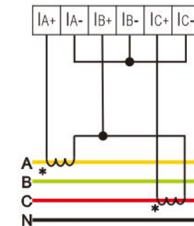
图 2.3.9 三相电流2CT接入
