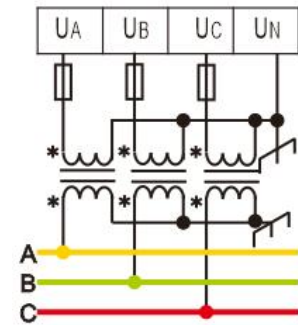
图 2.3.5 三相三线3PT接入
