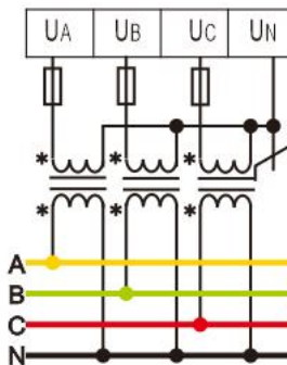
图 2.3.4 三相四线3PT接入
