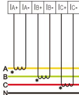
图 2.3.8 三相电流3CT接入
