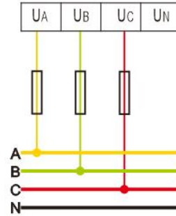
图 2.3.3 三相三线直接接入
