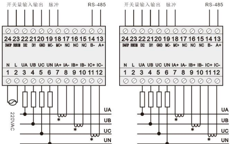
电源为独立端子供电型
